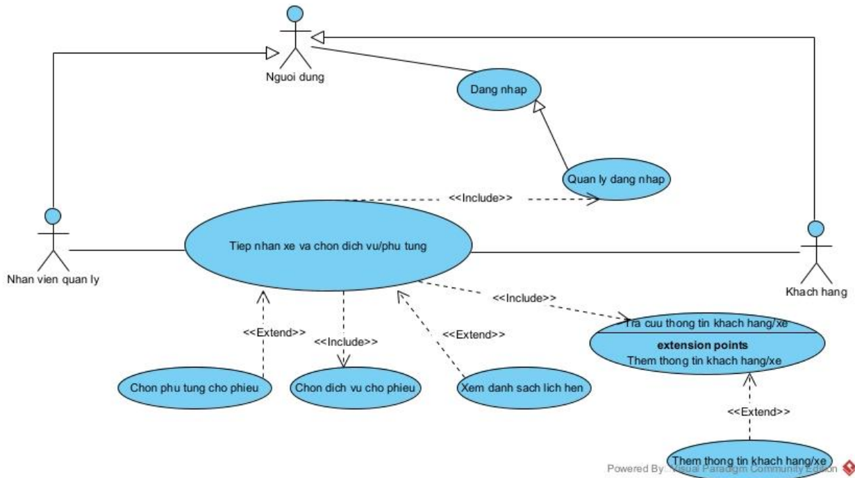
Hình 3.2 — Biểu đồ Use Case chi tiết: Tiếp nhận xe và chọn dịch vụ/phụ tùng
